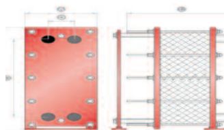
Dimensiones GL-13 (mm) A [330] B [775] C [590] D [135] L [de 6 a 30 placas] [470] L [de 32 a 60 placas] [570] L [de 62 a 92 placas] [670]
